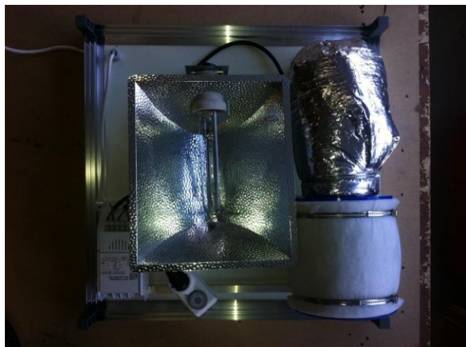
afbeelding 7 bovenplaat
