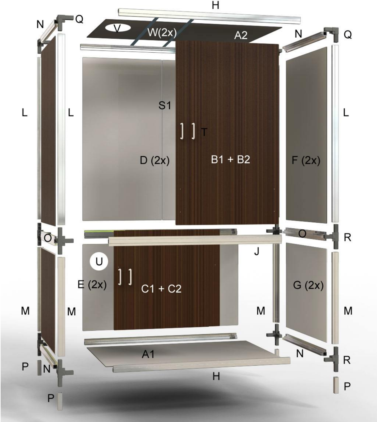
Afbeelding 1: samenstelling onderdelen kast G-kit Bonanza 250 (G-kit Bonanza 250 heeft 1 i.p.v 2 achterplaten)
